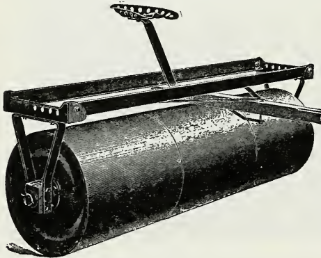
Fig. 130. A plain land roller.
