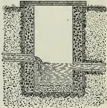
Fig. 64. A silt basin.
